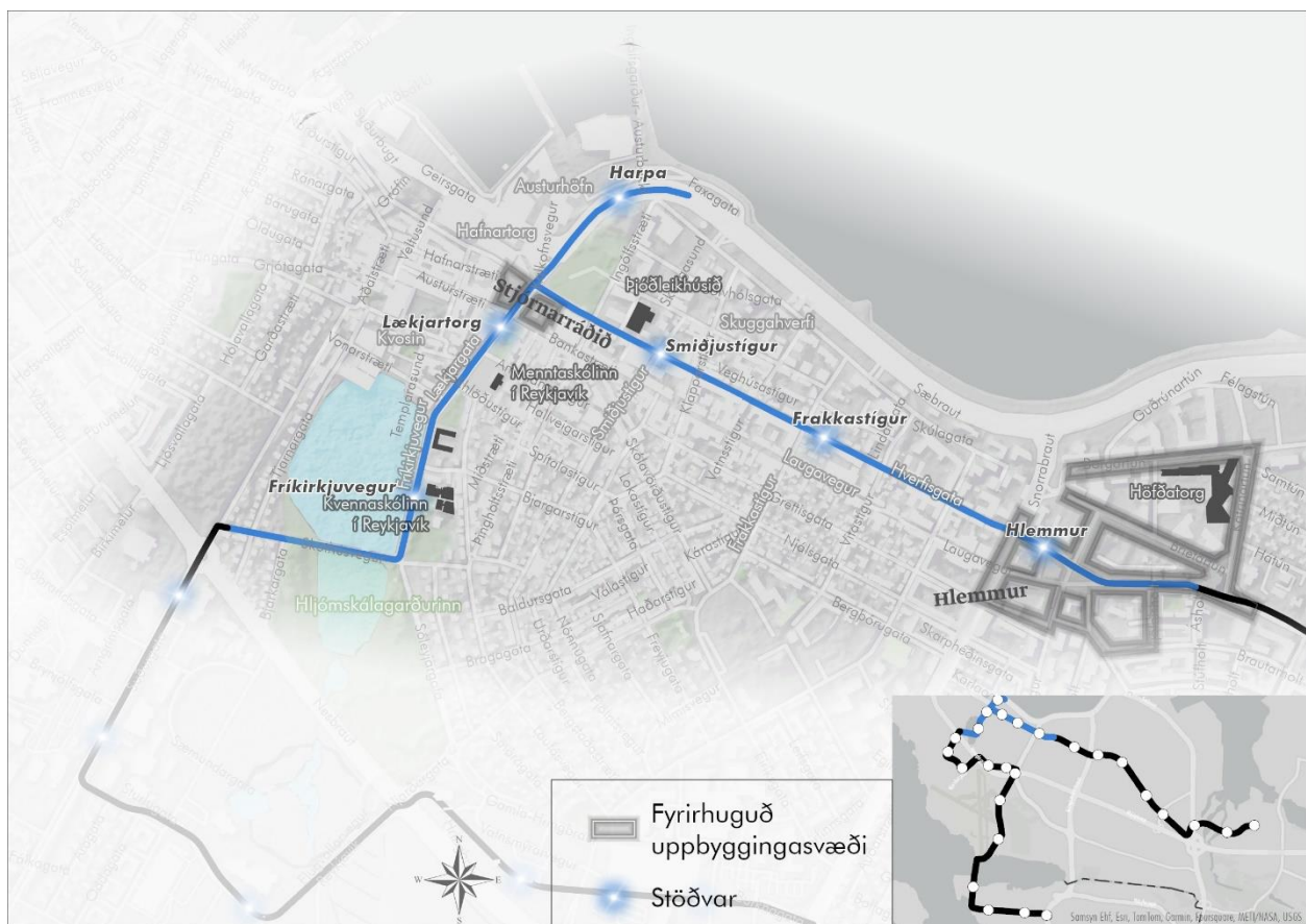
Mynd 5.20 Yfirlit yfir legg 140. Laugavegur – miðborg. Gráir rastar sýna aðliggjandi þróunarsvæði.
