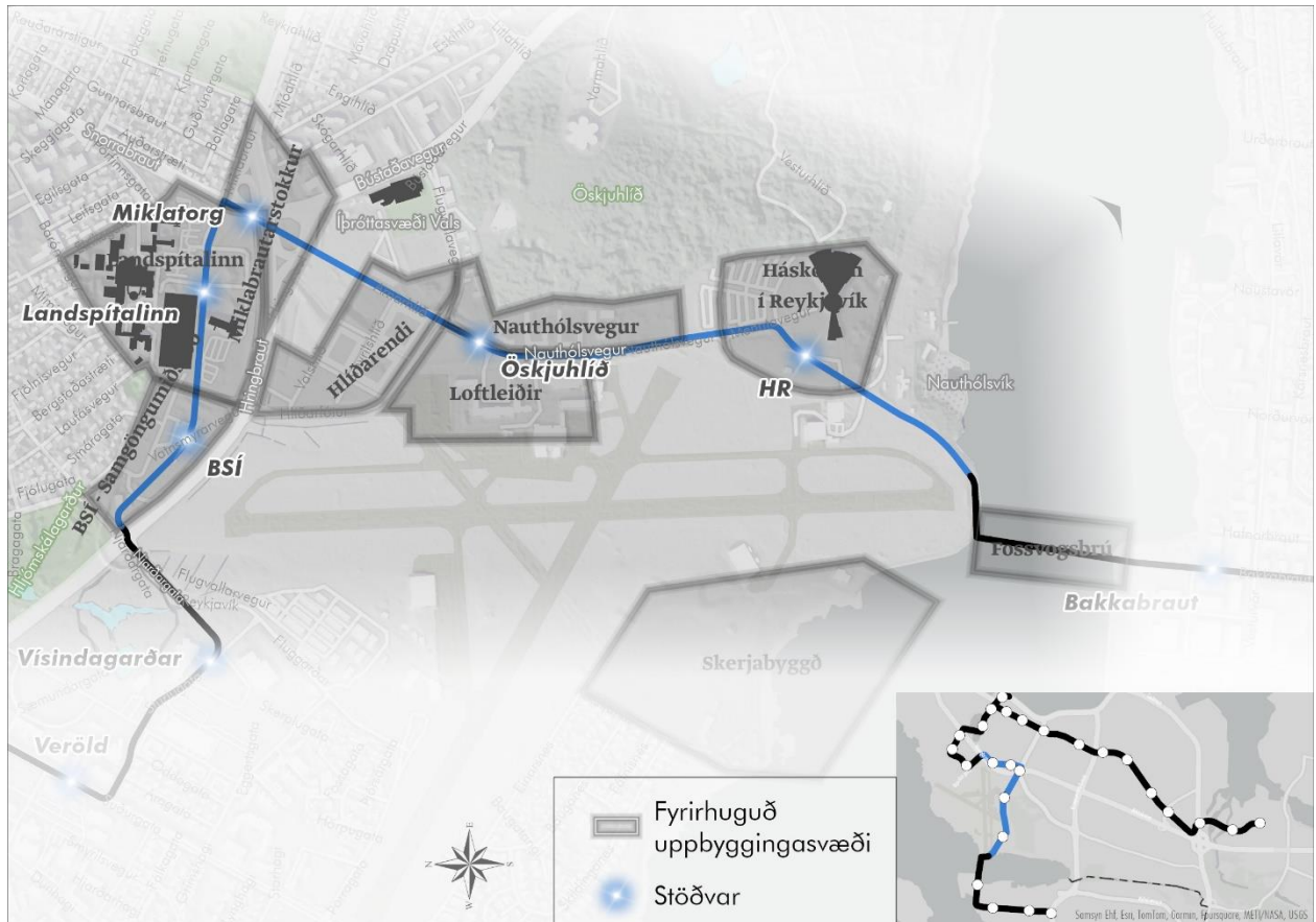
Mynd 5.35 Yfirlit yfir legg 160 Vatnsmýri-Fossvogsbrú. Gráir rastar sýna aðliggjandi þróunarsvæði.
