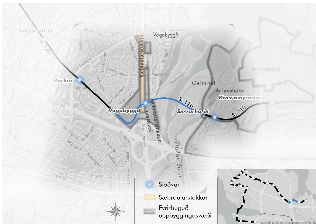
Mynd 5.12 Yfirlit yfir legg 120 Geirsnef og Vogabyggð.
