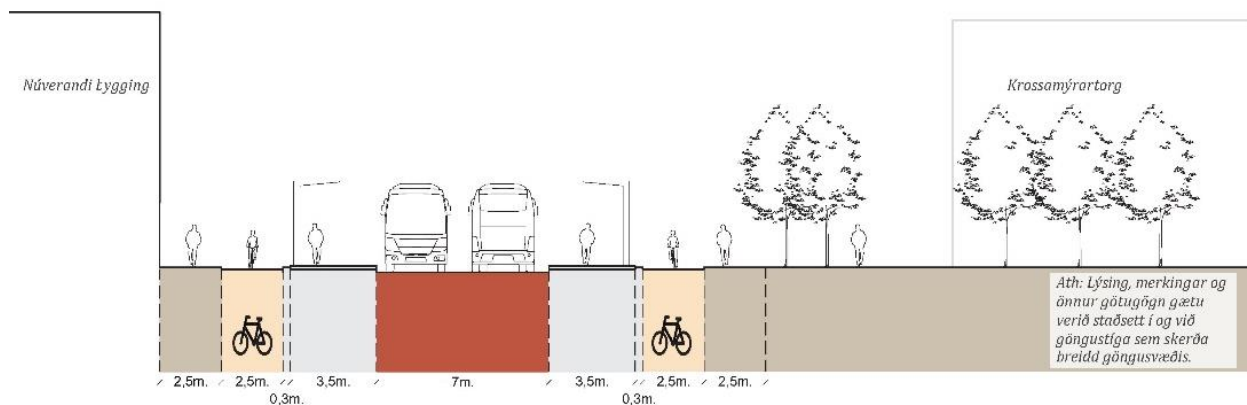
Mynd 5.11 Þversnið af Borgarlínustöð við Krossmýrartorg. Horft eftir Stórhöfða til vesturs í átt að gatnamótum við Breiðhöfða. (Snið AA – 1:2000) 20 .
