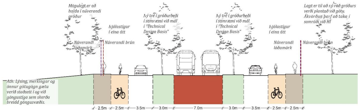
Mynd 5.30 Þversnið af ásýnd göturýmis á Suðurgötu framan við Hús íslenskunnar 35 , horft til suðvesturs.
