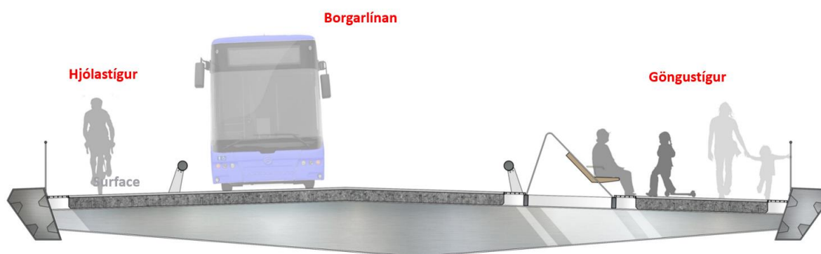
Mynd 5.42 Snið á brú yfir Fossvog, horft til suðurs. (Mynd: Efla 2023).
