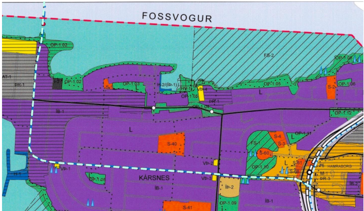
Mynd 7.33 Landnotkun í aðalskipulagi Kópavogs á Kársnesi. Borgarlínan skilgreind með ljósbílári punktalínu. Fjólublár stendur fyrir íbúðarbyggð, skástrikun fyrir þróunarsvæði, gulur fyrir miðsvæði, grár fyrir athafnasvæði og grænn fyrir opið svæði.
