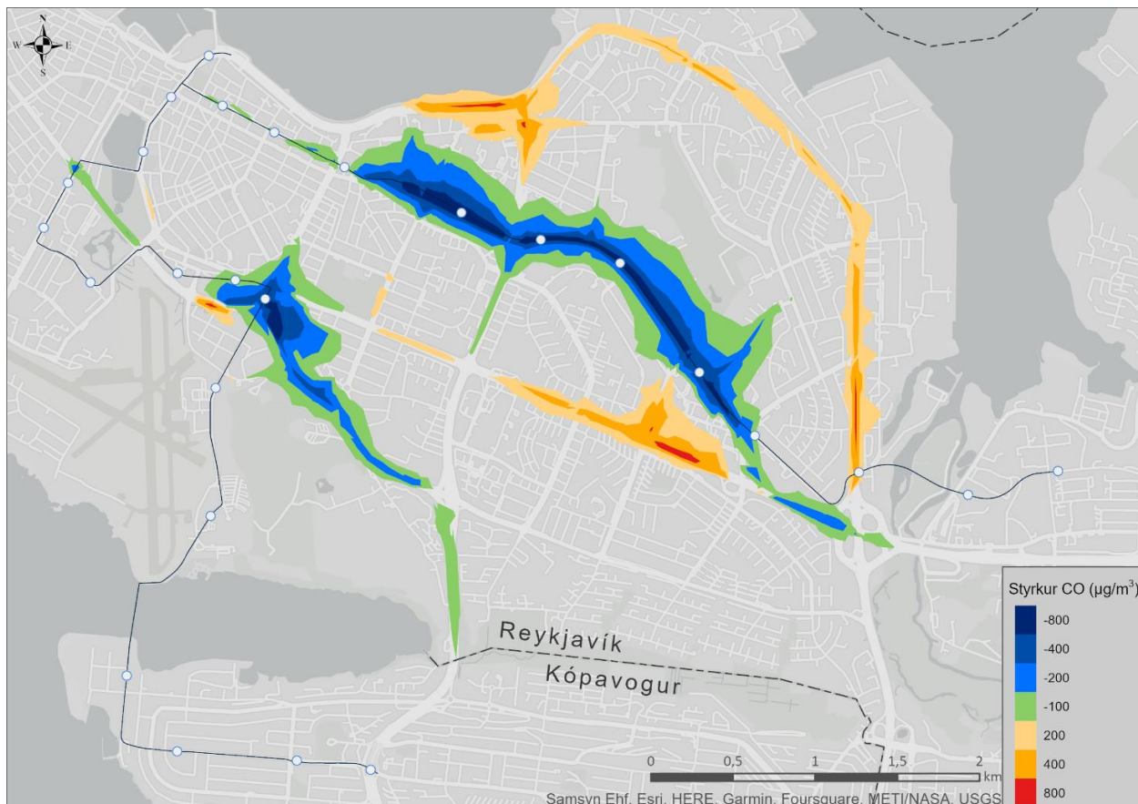
Mynd 7.15 Breyting á hæsta sólhrings gildi 8 klukkustunda hlaupandi meðaltals CO í framtíðartilviki með Borgarlínunni miðað við framtíðartilvik án Borgarlínunnar.
